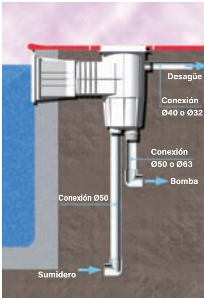
Instalación skimmer
