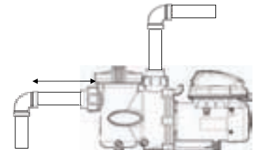
Correcto: Longitud del tubo de aspiración = 4 × diámetro del tubo (20 cm para 50 mm y 25 cm para 63 mm).
