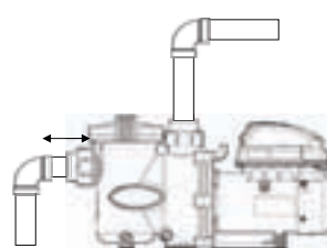
Incorrecto: Tubo de aspiración demasiado corto, riesgo de cavitación.
