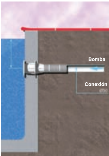
Instalación boquillas
