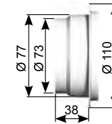
MAN 80 B integrado con la boca ref. BEIP 80
