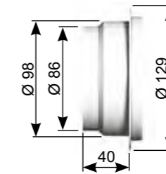
MAN 100 B integrado con la boca ref. BEIP 100
