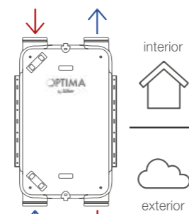
Modelo flujos de aire versión izquierda Ref: DFOPTIMAIBPL
