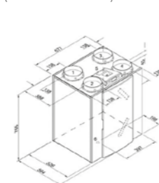
Siber® DF EXCELLENT 3/1 R (versión derecha)
