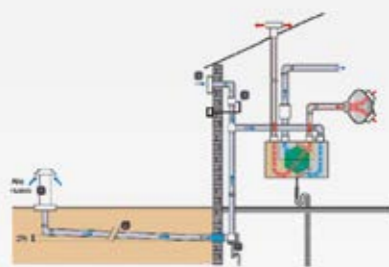
Registro en vivienda con sótano
