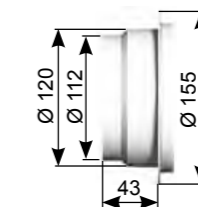
MAN 125 B integrado con la boca ref. BEIP 125
