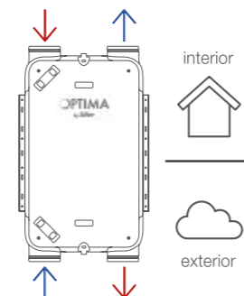
Modelo flujos de aire versión izquierda Ref: DFOPTIMA2BPL
