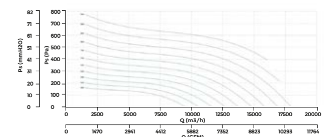
SIBERPARK CE 18/18 1,1kW
