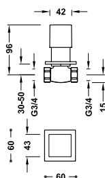
Llave de paso empotrada Conexión a rosca hembra: 3/4".
