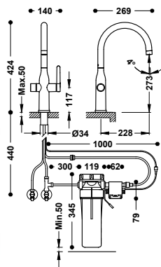
Grifo monomando de 2 vías para cocina, para agua de red y filtrada · Con sistema táctil para agua filtrada. · Incluye filtro para 6 meses (10.000 litros) de agua filtrada. · El filtro elimina bacterias, virus y metales pesados. · Latiguillos de alimentación flexibles G3/8.
