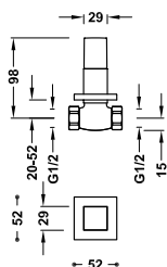
Llave de paso empotrada Conexión a rosca hembra: 1/2".
