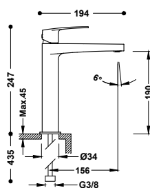
Grifo monomando alto ecoeficiente para lavabo Latiguillos de alimentación flexibles G3/8.
