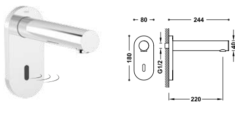
Grifo electrónico mural de 1 agua para lavabo Accionado mediante sensor de infrarrojos. La caja de la batería está localizada dentro del mismo caño. Conexión roscada macho de G1/2.
