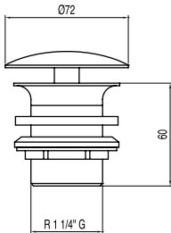
Válvula de desagüe siempre abierto para lavabo sin rebosadero Sin rebosadero. Tapón: Ø 72 mm.
