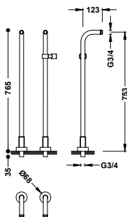
Tomas de agua acodadas de instalación a suelo para grifo de bañera 2 unidades con soporte fijo para ducha de mano.
