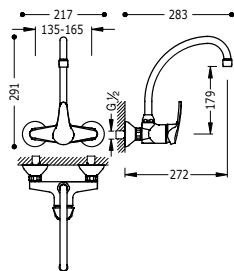
Grifo monomando mural para cocina Con caño superior. Distancia a pared: 272 mm.
