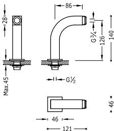
Tomas de agua acodadas de instalación a borde bañera para grifo de bañera 2 unidades con silenciador.
