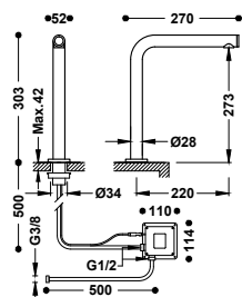
Grifo electrónico de 1 agua para cocina Sistema sensible al tacto Touch-tres. Con latiguillo de alimentación flexible G3/8.
