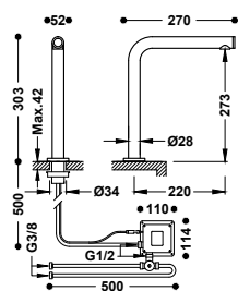
Grifo electrónico con sistema premezclador para cocina Sistema sensible al tacto Touch-tres. Incluye una válvula mezcladora de 2 aguas con tubos flexibles. Con latiguillos de alimentación flexibles G3/8.
