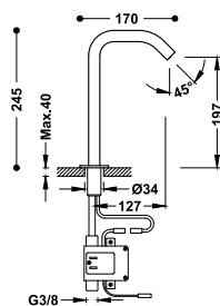
Grifo electrónico de 1 agua para lavabo Accionado mediante sensor de infrarrojos.
