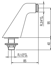
Tomas de agua acodadas de instalación a borde bañera para grifo de bañera 2 unidades con silenciador.
