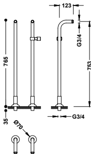
Tomas de agua acodadas de instalación a suelo para grifo de bañera 2 columnas verticales de alimentación de agua a suelo.
