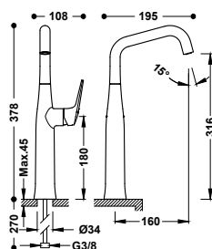
Grifo monomando XL con maneta lateral para lavabo Latiguillos de alimentación flexibles G3/8.
