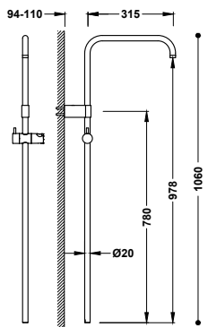
Barra de ducha larga adaptable a grifo termostático mural con conexión compatible
