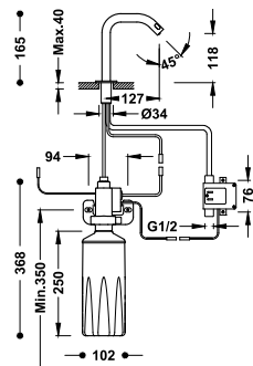
Grifo electrónico de 1 agua con dispensador de jabón automático para lavabo
