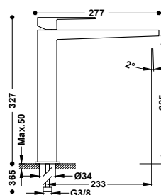
Grifo monomando XL para lavabo Latiguillos de alimentación flexibles G3/8.
