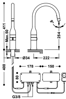
Grifo electrónico para cocina
