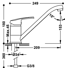
Grifo monomando para cocina Con latiguillos de alimentación flexibles G3/8.
