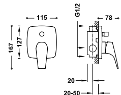
Grifo monomando empotrado de 2 vías para bañera y ducha Cuerpo empotrado incluido. Inversor de 2 vías.
