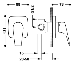
Grifo monomando empotrado de 1 vía para ducha Cuerpo empotrado incluido.
