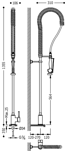
Grifo monomando con ducha extraíble para cocina industrial
