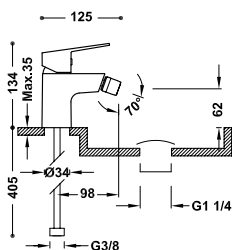
Grifo monomando para bidé con válvula desagüe Click-clack Latiguillos de alimentación flexibles G3/8.
