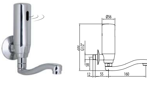
Grifo electrónico mural de 1 agua para lavabo Accionado mediante sensor de infrarrojos.
