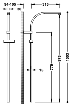
Barra de ducha larga adaptable a grifo termostático mural con conexión compatible
