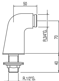
Tomas de agua acodadas de instalación a borde bañera para grifo de bañera 2 unidades con silenciador.
