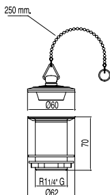
Válvula de desagüe con tapón y cadenilla para lavabo sin rebosadero Cadenilla de 250 mm.
