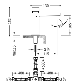
Grifo temporizado de 1 agua con sistema premezclador para lavabo Cierre automático: 6 seg. Incluye una válvula mezcladora de 2 aguas con tubos flexibles. Caudal: 0,7 l x ciclo.
