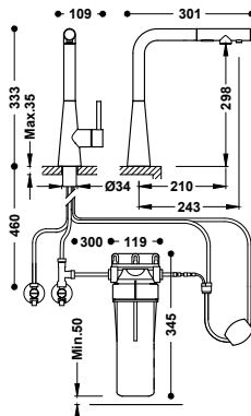
Grifo monomando de 2 vías con caño extraíble para cocina, para agua de red y filtrada · Con pulsador para agua filtrada. · Material: Acero inoxidable. · Incluye filtro para 6 meses (10.000 litros) de agua filtrada. · El filtro elimina bacterias, virus y metales pesados. · Latiguillos de alimentación flexibles G3/8.
