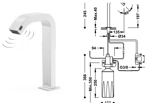
Grifo electrónico de 1 agua con dispensador de jabón automático para lavabo Accionado mediante sensor de infrarrojos. Capacidad del depósito de jabón: 1600 ml.
