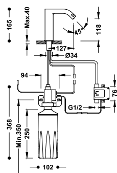
Grifo electrónico de 1 agua con dispensador de jabón automático para lavabo
