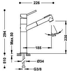
Grifo monomando con caño extraíble con 2 funciones para cocina Con latiguillos de alimentación flexibles G3/8.
