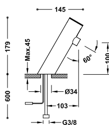
Grifo electrónico de 1 agua para lavabo Accionado mediante sensor de infrarrojos. Caudal: 6 l/min.
