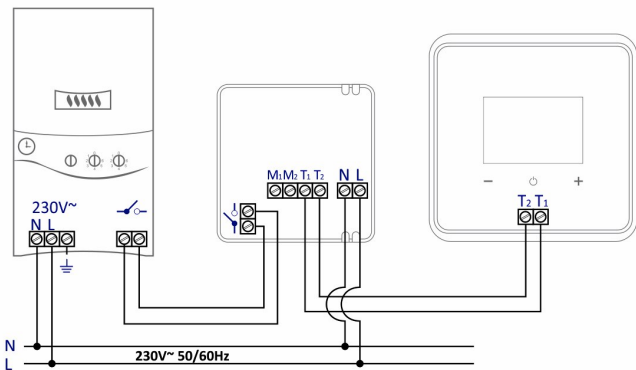
Caldera combi acción Todo/Nada
