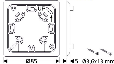
Placa TA (placa montaje + tornillos)
