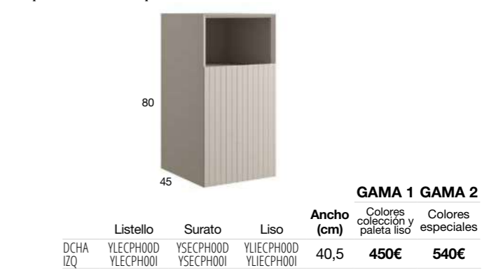
coqueta 1 hueco 1 puerta
