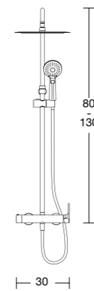
Fonte columna ducha monomando
