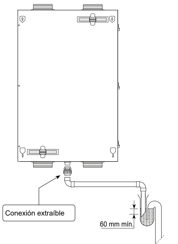
Desagüe de condensación para montaje en pared CWL - F - 200 Excellent (VHZ)
