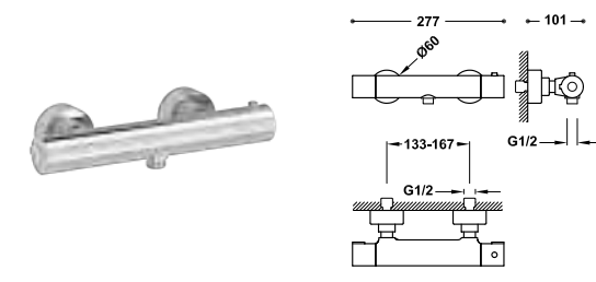
Grifo termostático mural para ducha Sin complementos.
