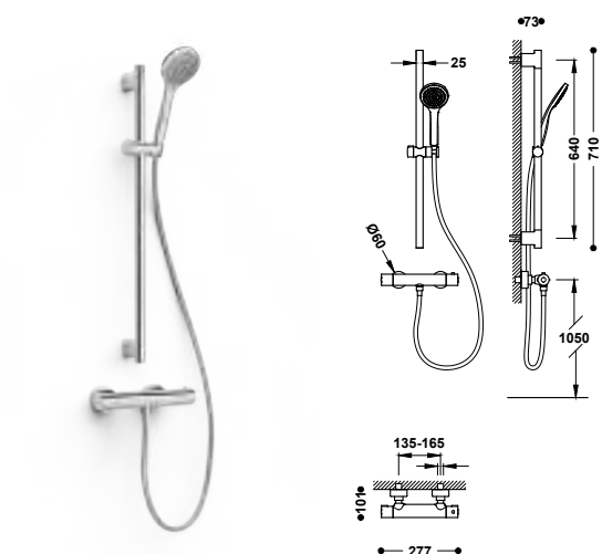
Kit de grifo termostático mural para ducha
