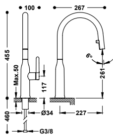
Grifo monomando con caño extraíble con 2 tipos de chorro para cocina Con flexo retráctil de poliamida trenzada. Con latiguillos de alimentación flexibles G3/8.
