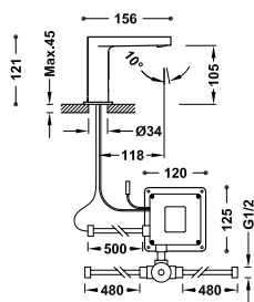
Grifo electrónico con sistema premezclador para lavabo Accionado mediante sensor de infrarrojos. Incluye una válvula mezcladora de 2 aguas con tubos flexibles.
