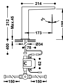
Grifo electrónico con sistema premezclador para lavabo Accionado mediante sensor de infrarrojos. Incluye una válvula mezcladora de 2 aguas con tubos flexibles.
