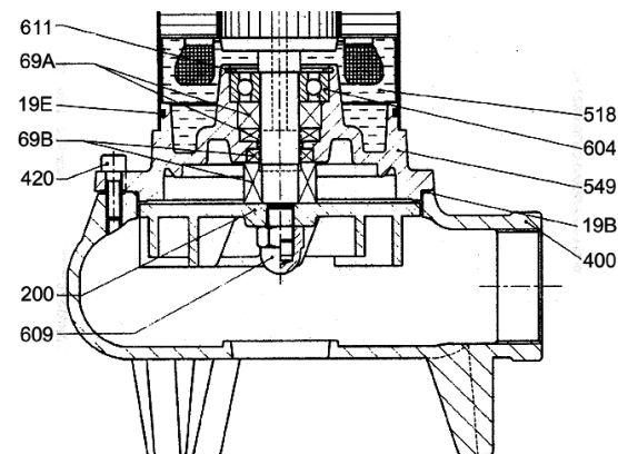
DESPIECE B3
