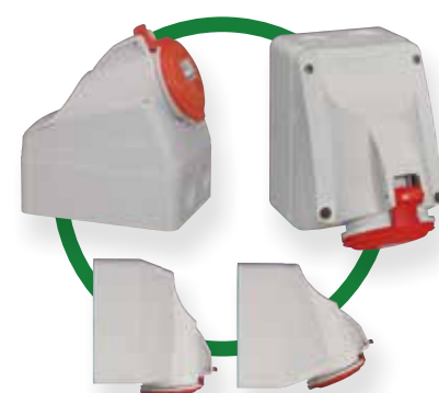
Base mural de superficie 3P+T - 32A IP44 - 380/415 V Ref. 090161
