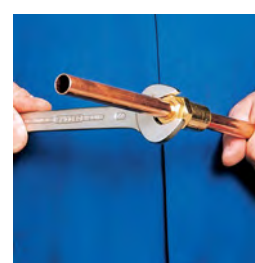
7. Apretar con una llave inglesa. 7. Apertar com uma chave inglesa.
