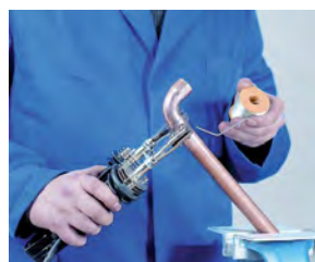
5. Aplicación de la soldadura 5. Aplicação da soldadura
