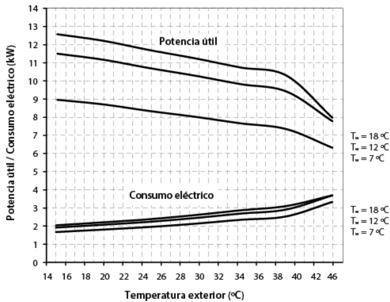
Curvas de prestaciones en enfriamiento Dual Clima 12HT
