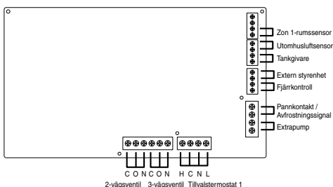
2-vägsventil 3-vägsventil Tillvalstermostat 1
