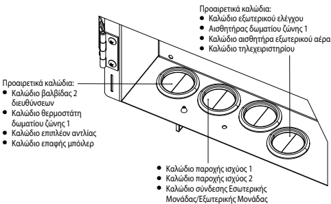
Τρόπος οδήγησης των προαιρετικών καλωδίων και του καλωδίου παροχής ισχύος (προβολή χωρίς εσωτερικές καλωδίώσεις)
