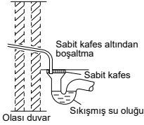
Boşaltma hortumunun dışarıya yönlendirilmesinin resmi
