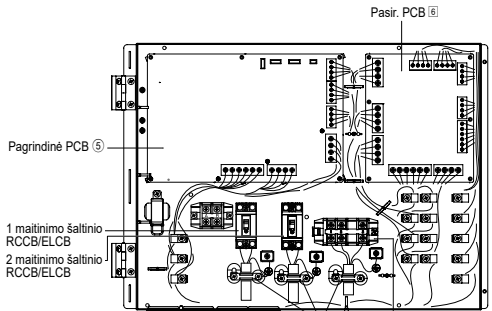
Kaip pravesti pasirinktinius kabelius ir maitinimo šaltinio kabelį (vaizdas be vidinių laidų)
