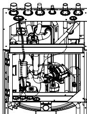
Καλωδίωση για τον "ΣΥΝΔΥΑΣΜΟ-1"
