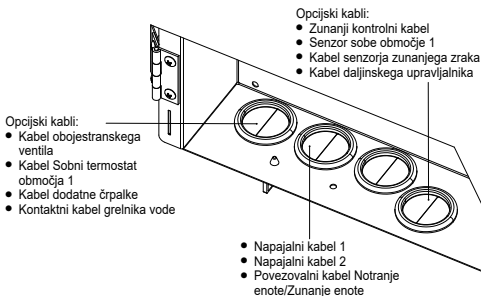
Kako voditi opcijske kable in napajalni kabel (pogled brez notranje napeljave)
