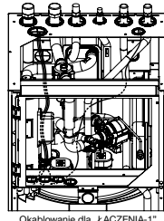
Okablowanie dla „ŁĄCZENIA-1”
