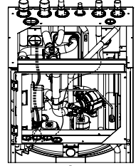
YHDISTELMÄ-2-n johdotus
