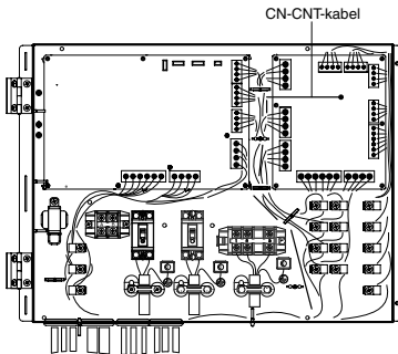
Med tilläggskort
