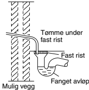
Illustrasjon av føring av tømmeslange ut
