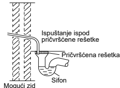
Ilustracija vođenja odvodnog crijeva na izvan prostorije
