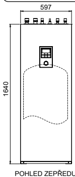
POHLED ZEPŘEDU
