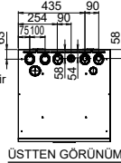
ÜSTTEN GÖRÜNÜM
