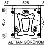
ALTTAN GÖRÜNÜM
