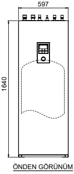
ÖNDEN GÖRÜNÜM
