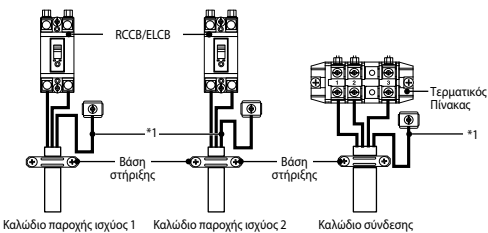
Καλώδιο παροχής ισχύος 1 Καλώδιο παροχής ισχύος 2 Καλώδιο σύνδεσης
