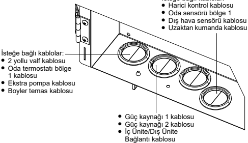
İsteğe bağlı kabloların ve güç kaynağı kablosunun yönlendirilmesi (dahili tesisatı olmadan görünüm)
