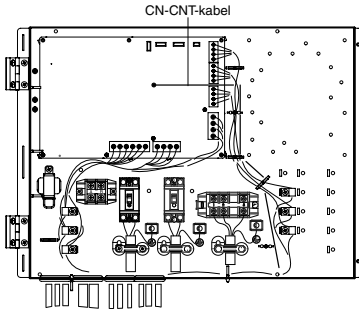
Utan tilläggskort
