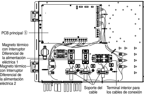
Cómo guiar los cables y el cableado de alimentación de la instalación (vista sin el cableado interno)
