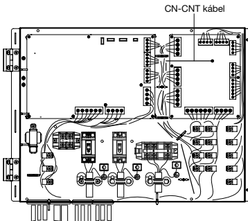
Opcionális panel-val
