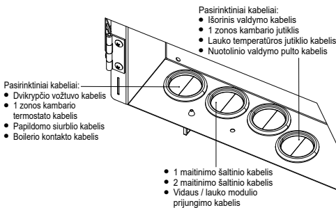
Kaip pravesti pasirinktinius kabelius ir maitinimo šaltinio kabelį (vaizdas be vidinių laidų)
