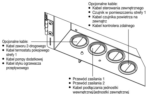
Prowadzenie kabli opcjonalnych przewodu zasilającego (widok bez okablowania wewnętrznego)
