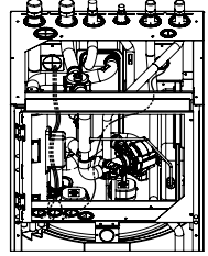
Verkabelung für „KOMBIKATION-2“
