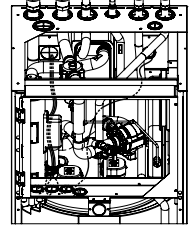
„2. KOMBINÁCIÓ” vezetékvezetése
