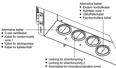
Hvordan trekke de ekstra kablene og strømledningen (vist uten intern kabling)
