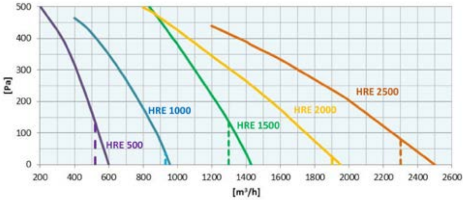
CURVA PRESION DISPONIBLE - CAUDAL FILTRA F7 EN AIRE NUEVO
